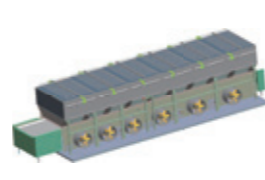
Fluidized IQF 流态化速冻机
